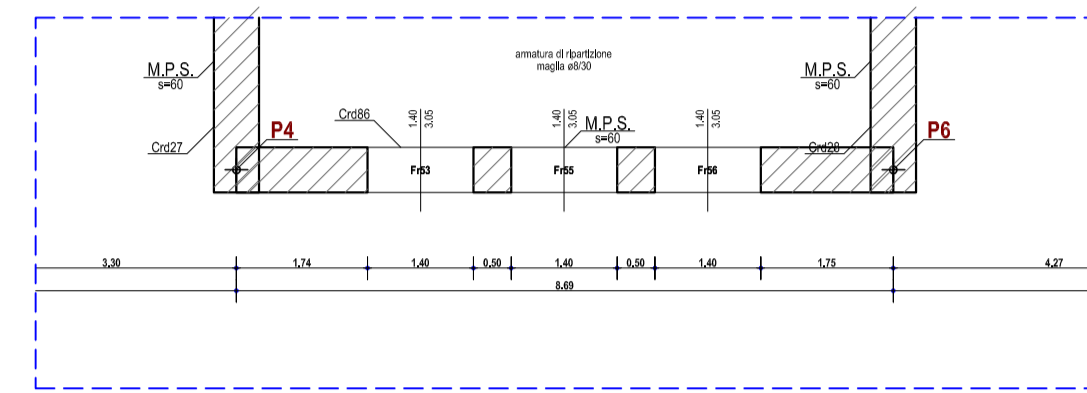
Area di intervento stato attuale
