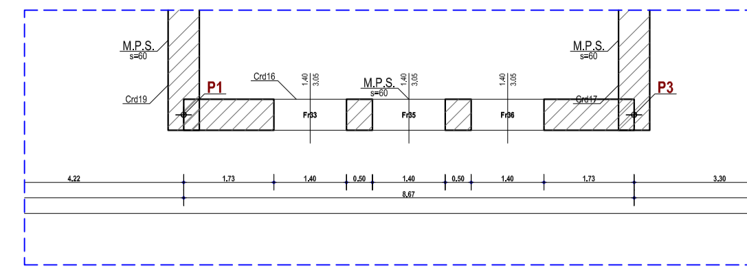
Area di intervento stato attuale
