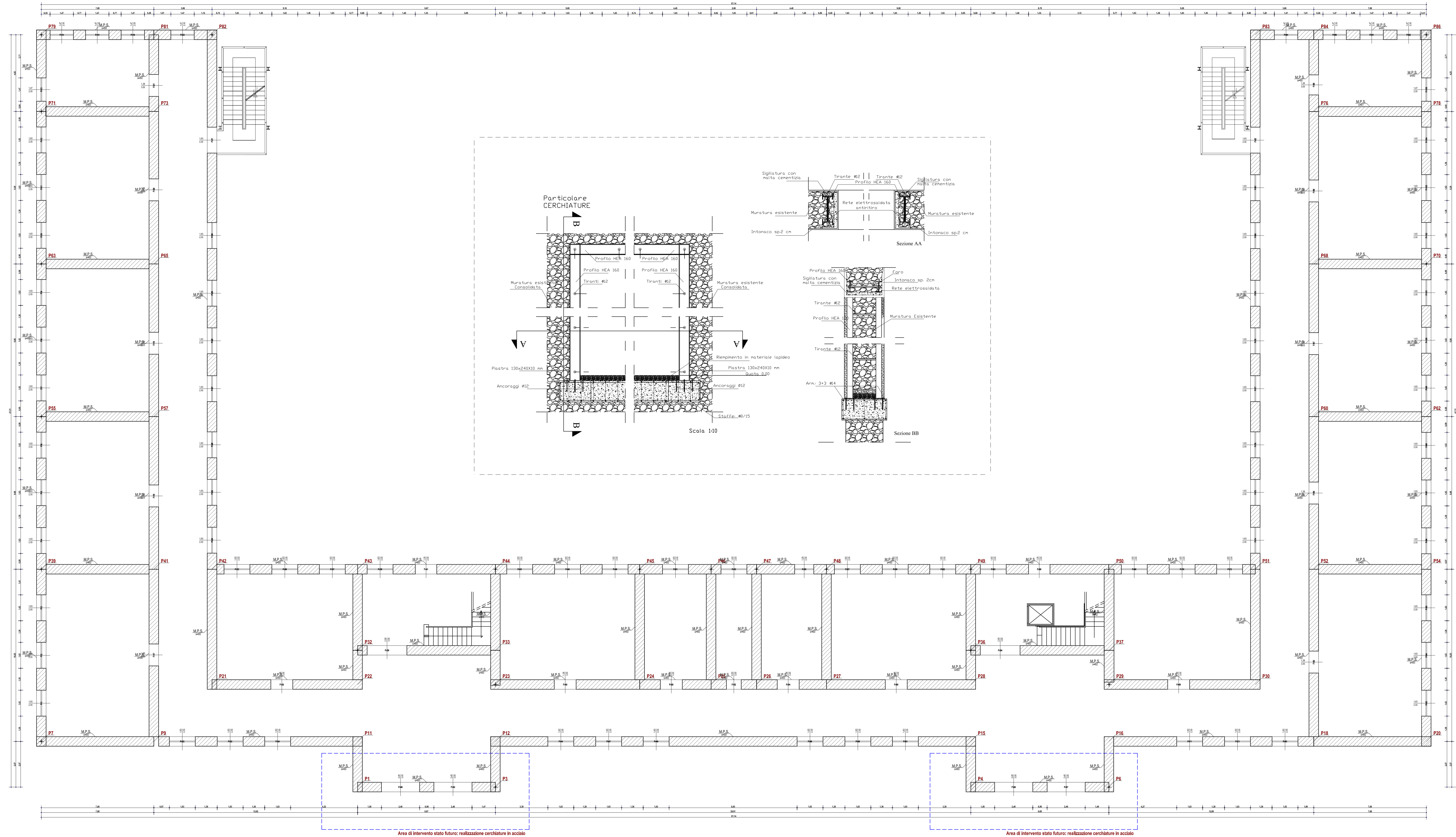
Area di intervento stato futuro: realizzazione cerchiature in acciaio
